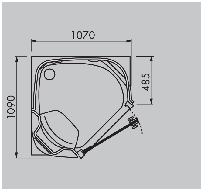
Bovenaanzicht hoekinbouw (in mm)
