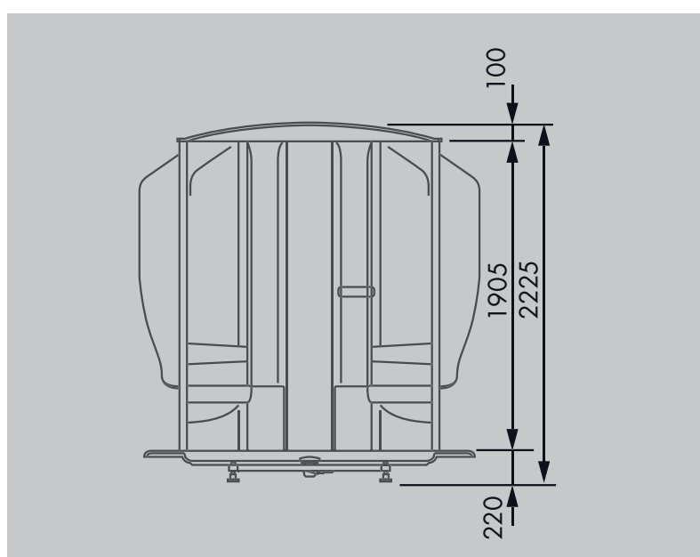
Vooraanzicht (in mm)
