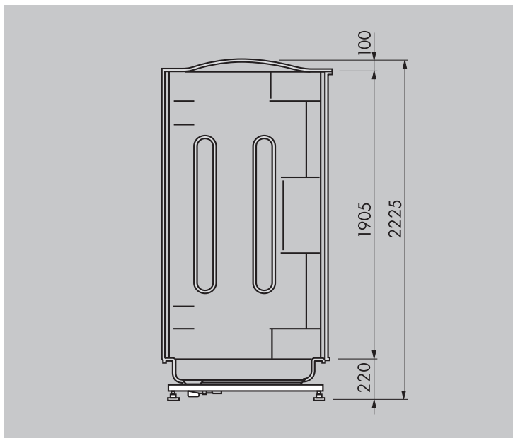
Vooraanzicht (in mm)
