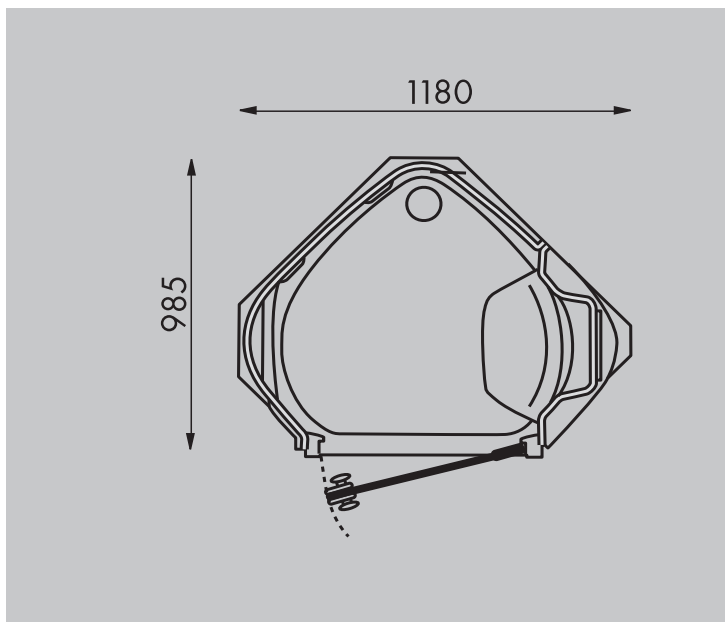
Bovenaanzicht wandinbouw (in mm)
