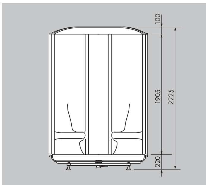
Vooraanzicht (in mm)
