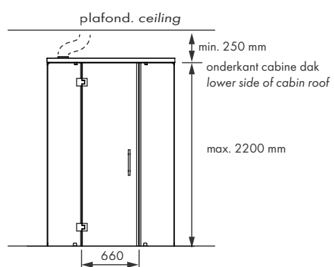
VOORBEELD INSTALLATIE: CABINEDAK GEKOPPELD AAN GLASFRONT.
