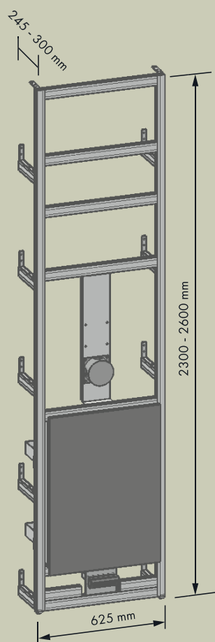
BackWall zonder bouwplaat. Maximale dikte van afwerking incl. tegel is 30 mm.
