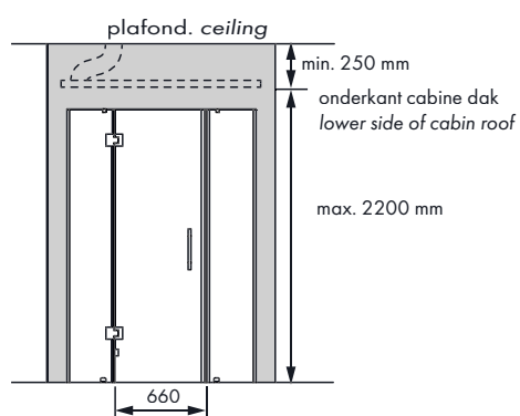
VOORBEELD INSTALLATIE: INGEBOUWD CABINEDAK.
