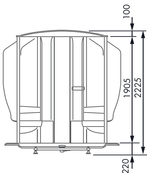
Vooraanzicht (in mm)
