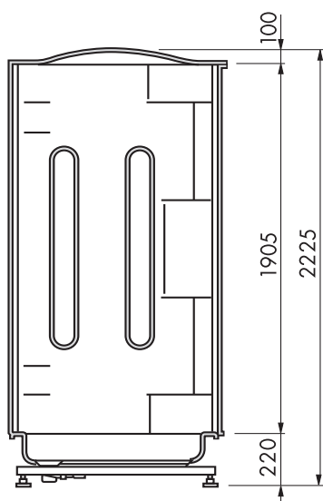
Voorraanzicht (in mm)
