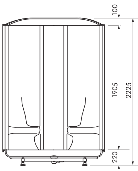
Vooraanzicht (in mm)
