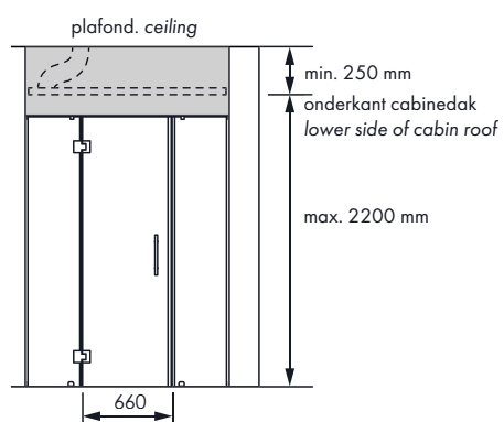
VOORBEELD INSTALLATIE: INGEBOUWD CABINEDAK.
