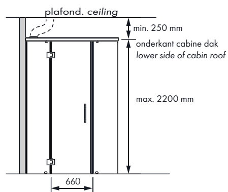
VOORBEELD INSTALLATIE: CABINEDAK GEKOPPELD AAN GLASFRONT.
