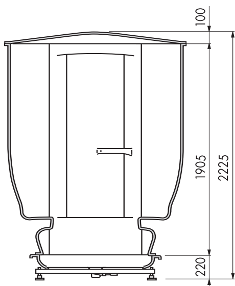
Voor aanzicht (in mm)
